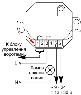
Рисунок 3. Схема подключения к лампе накаливания и блоку управления автоматикой
