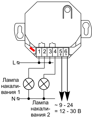
Рисунок 2. Схема подключения к двум лампам накаливания
